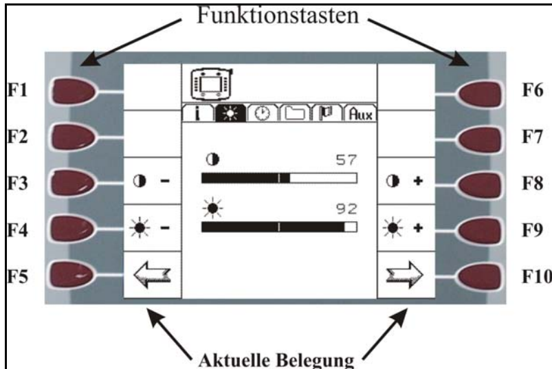
Rys. -17: Przyciski funkcyjne - przykład: „Ustawienia ekranu“
